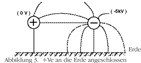
Abbildung 3. +Ve an die Erde angeschlossen
