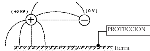
Figura 2. Protección a tierra
