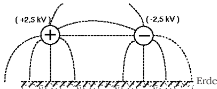
Abbildung 1. Erdungsprüfung
